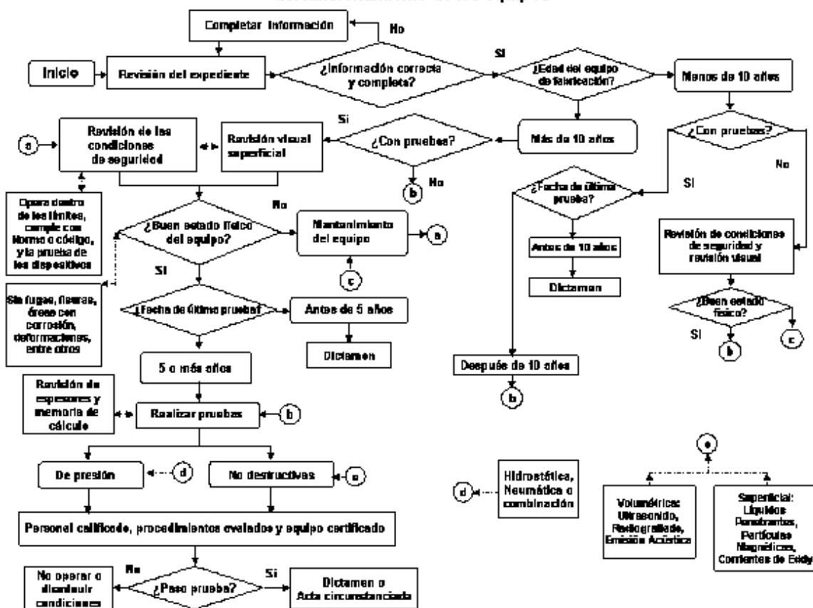
Diagrama 1 Análisis de las condiciones de seguridad del funcionamiento de los equipos
